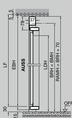
Sezione verticale portone senza battuta inferiore
