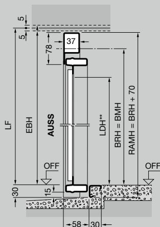
Sezione verticale portone con battuta inferiore
